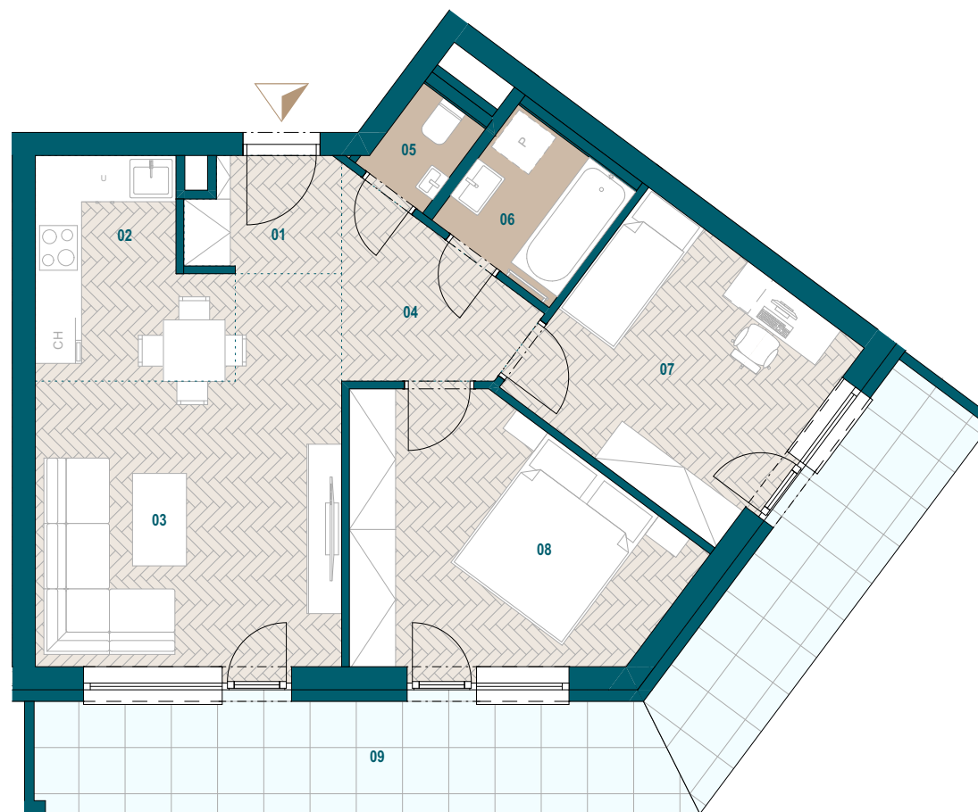
4. nadzemné podlažie
